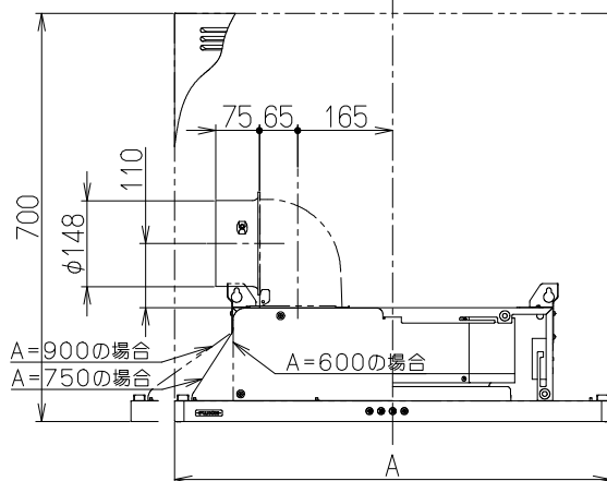
側方排気の場合 (別売L形ダクト使用時)
