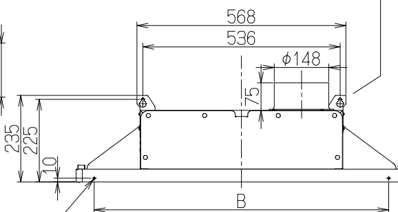
後方排気の場合 (別売L形ダクト使用時)
